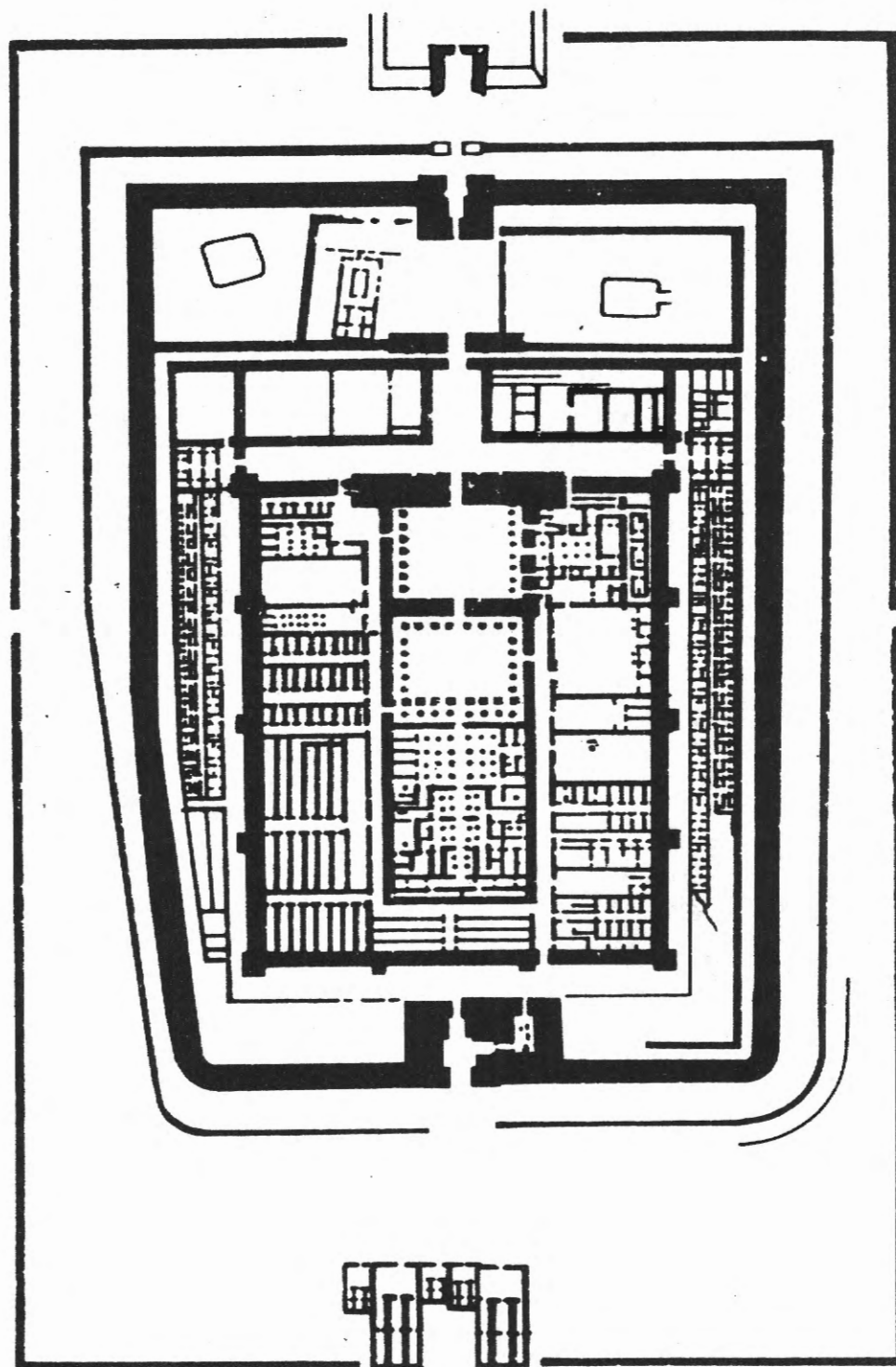
FIG. 10.—Templo funerario de Ramsés III en Medinet Habu (redibujado de Vandier 1955, Tomo II, p. 751, fig. 373).
